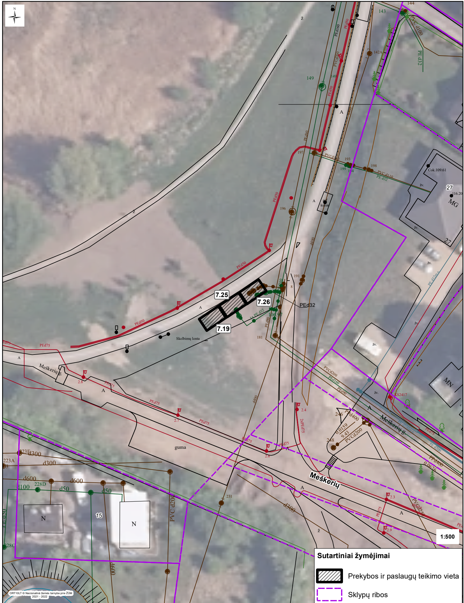
Talkšos ežero pakrantės (take nuo Frenkelių g. 17 link Tinklų g.) schema M 1:500
