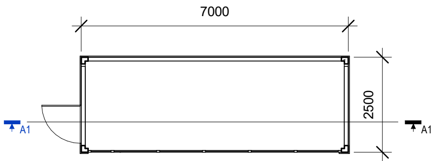
Kiosko planas 1 : 100
