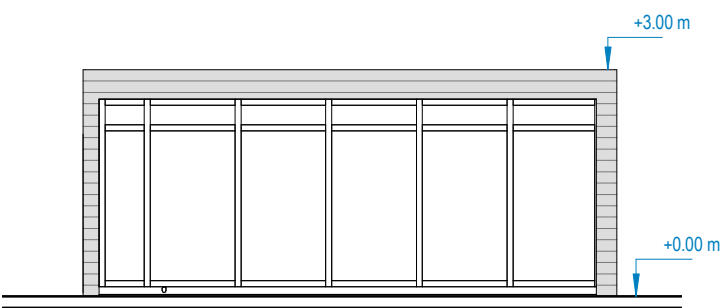
Kiosko fasadas 1 : 100
