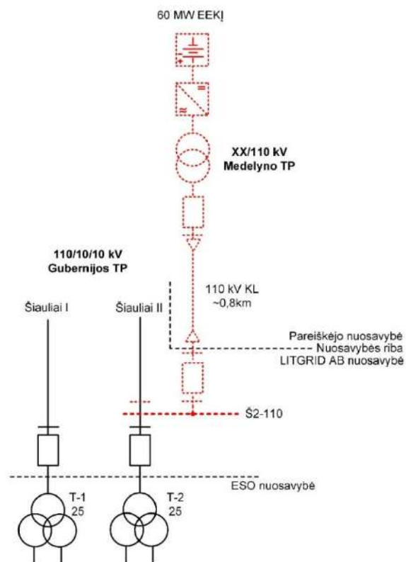
Pav. 5. Planuojamo BEKS prijungimo prie elektros perdavimo tinklo principinė schema.
