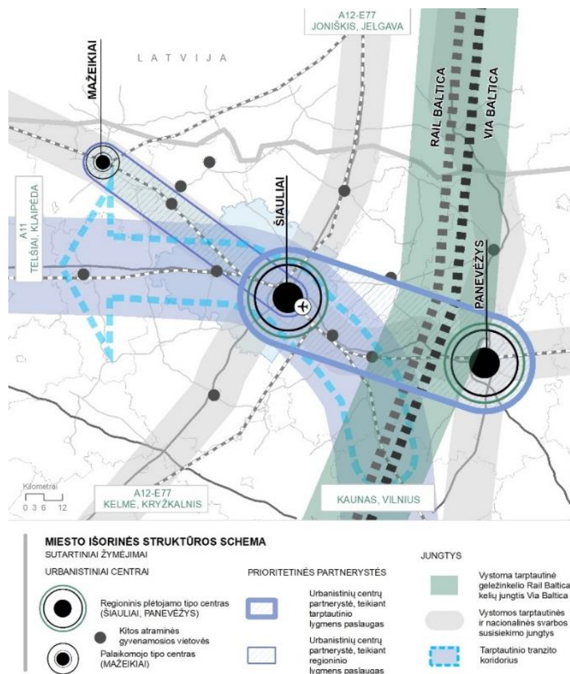
2.1.5.13 pav. Miesto išorės struktūros schema. IV alternatyva.
