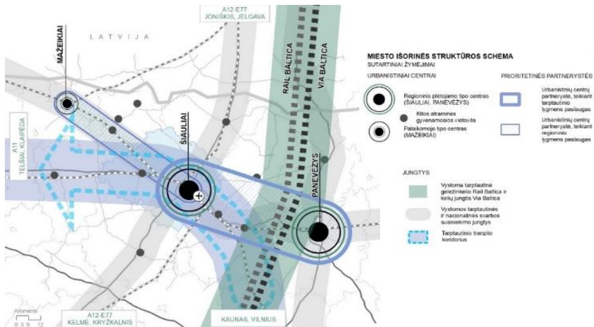
2.1.5.5 pav. Miesto išorės struktūros schema. II alternatyva.
